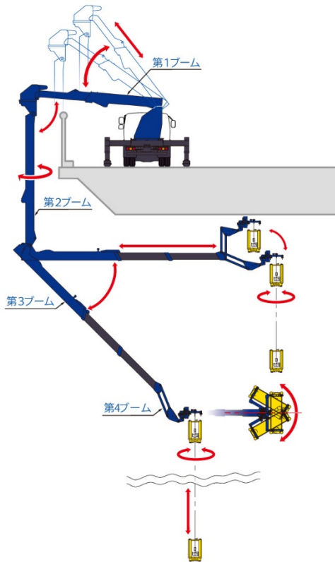
▲ 橋梁下部64.5mまでアクセス可能なゴンドラ車
